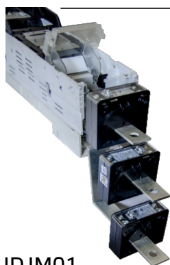
IDJM01 Комплект накладок для установки трансформаторов тока для VFSD-630, VFSD-400
